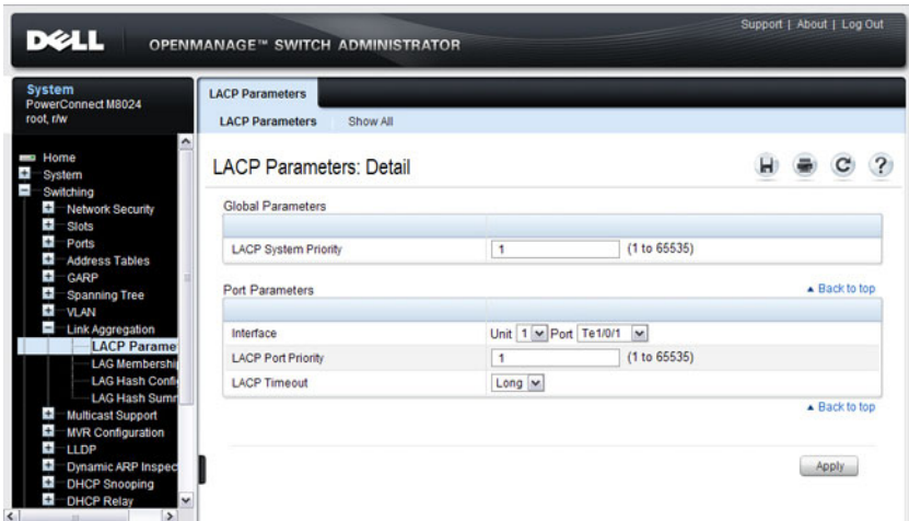
Figure 28-3. LACP Parameters
